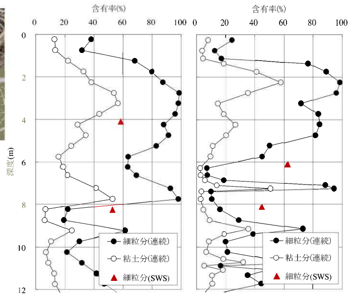
(a)地点1 (b)地点3 図-4 土質(粒度)試験結果
