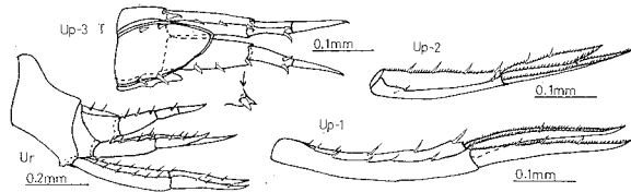
Fig. 278. Stenothoe valida Dana. Male, 2.5 mm.
