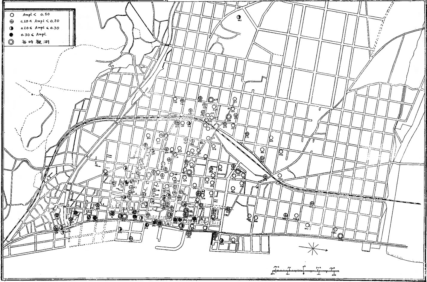
第2圖 別府温泉感潮度分布
