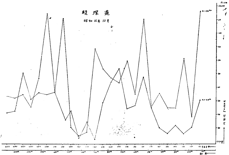
第6圖 的石一殿塚道に沿ふ比抵抗水平分布
