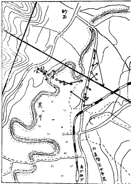
第8圖 赤水一的石道附近地電位傾度分布
