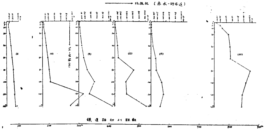
第5圖 赤水一的石道路上6點の比抵抗垂直分布
