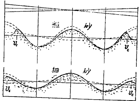
第 6 圖 掃流二次作用による砂堆の形状
