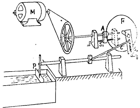
第 1 圖 沙堆及び沙澱實驗裝置
