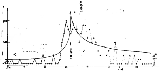
第 4 圖 阿蘇間歇泉昭和18年6月13日12時、噴騰における噴出頻度観測値 (毎分) 實線は計算値、破線は開口期、點線は噴出期 (始12時7分、終20時27分)
