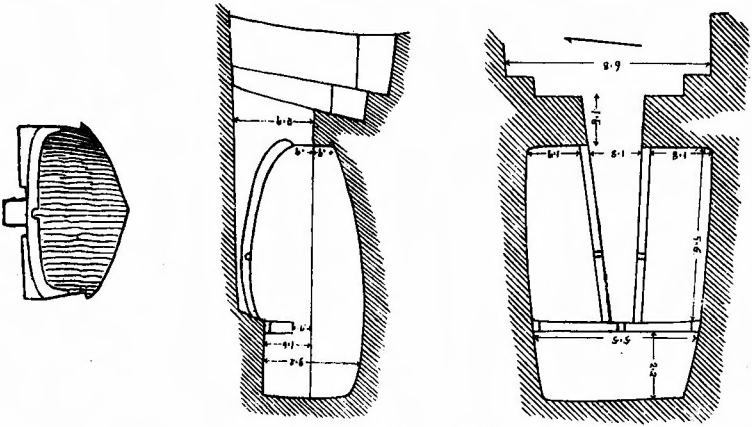
合上第廿一號模範之全形及剖面圖
