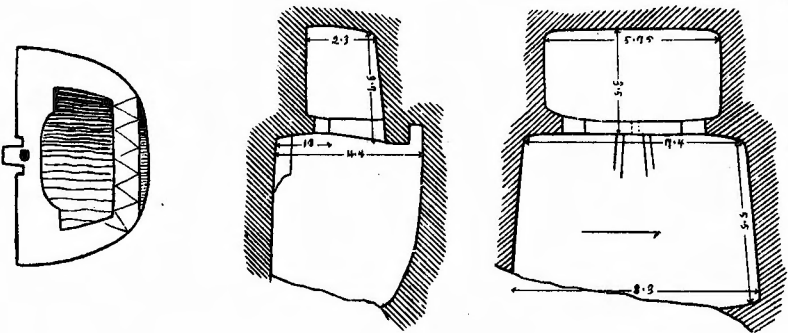
肥後國三木郡五曾村大子屋第二十七號模範之全形及剖面圖
