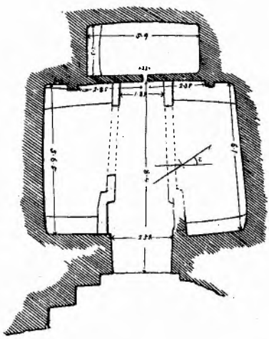
肥後國玉名郡石賀村石賀橋穴第八號穴 大正三年三月再測
