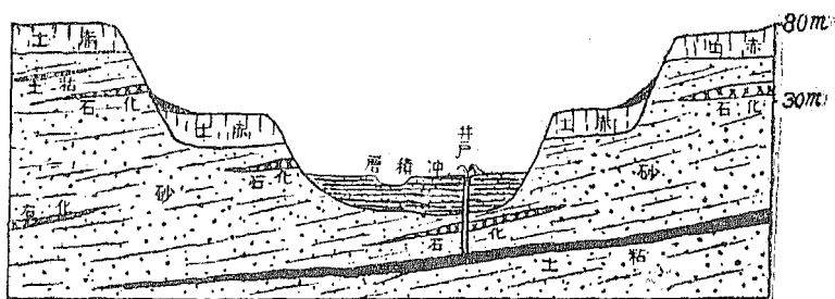
千葉縣原市郡東村附近理想断面圖
