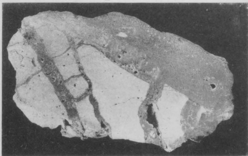
黒鐵々脈に貫かれた石英粗面岩 小坂鑛山鑛床の母岩
