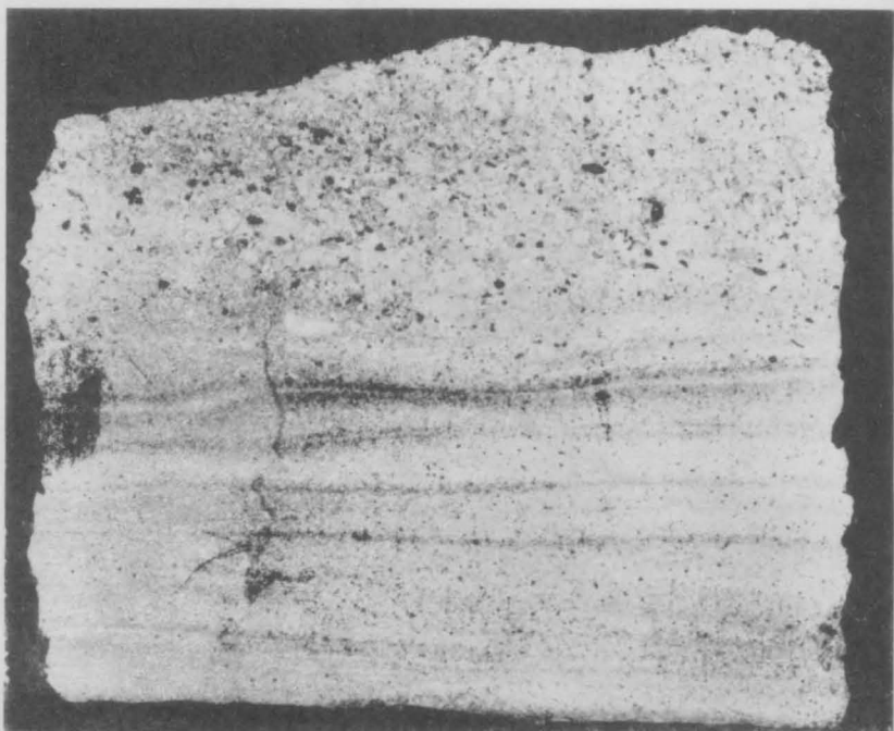
鐵化を免れた角礫岩層の一部
