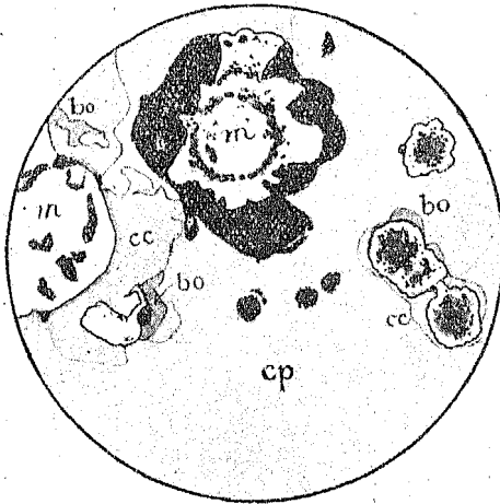
圖二第 黃銅鑛(cp)中に生ぜざる銅鑛(cc)及び斑銅鑛(bo)の白鐵鑛(m)に伴ふな態を示す(約二百倍) (主は部色黒しと白鐵鑛の欠損部)
