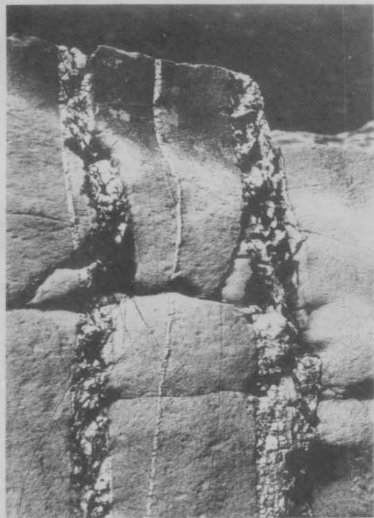
第三圖 蛇石第一脈Aノ一部ヲ明ニセルモノ横ノ節理モ明カナリ(高さ約八〇糎)
