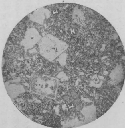
PL. 斜長石 H. 紫蘇輝石 A. 普通輝石 M. 磁鐵鑛
