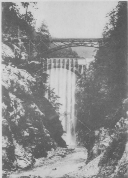
第二圖 跡曳水路橋
