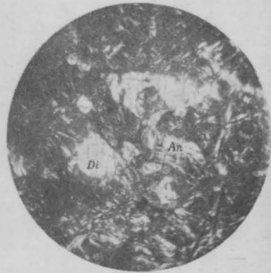
大日向村都澤の黑色緻密蛇紋岩(十字ニコル) Di 異剝石 An 板温石
