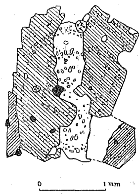
包裹物帶が斜長石(p), 輝石(a), 紫蘇輝石(h), に亘つて居る例 (No. 341089, II, 24の略圖)
