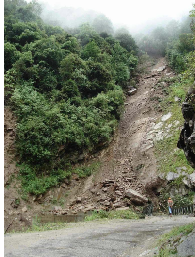
写真2 インド北東部、アルナチャル・プラデシュ州、タワン地域で観察された斜面崩壊 (2007年7月23日撮影)
