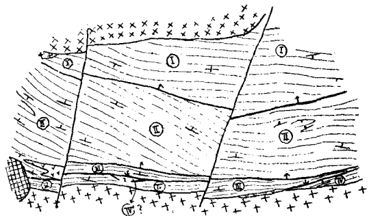
第3圖 夜久野附近地質構造概念圖 Schematic map of the geological str.
