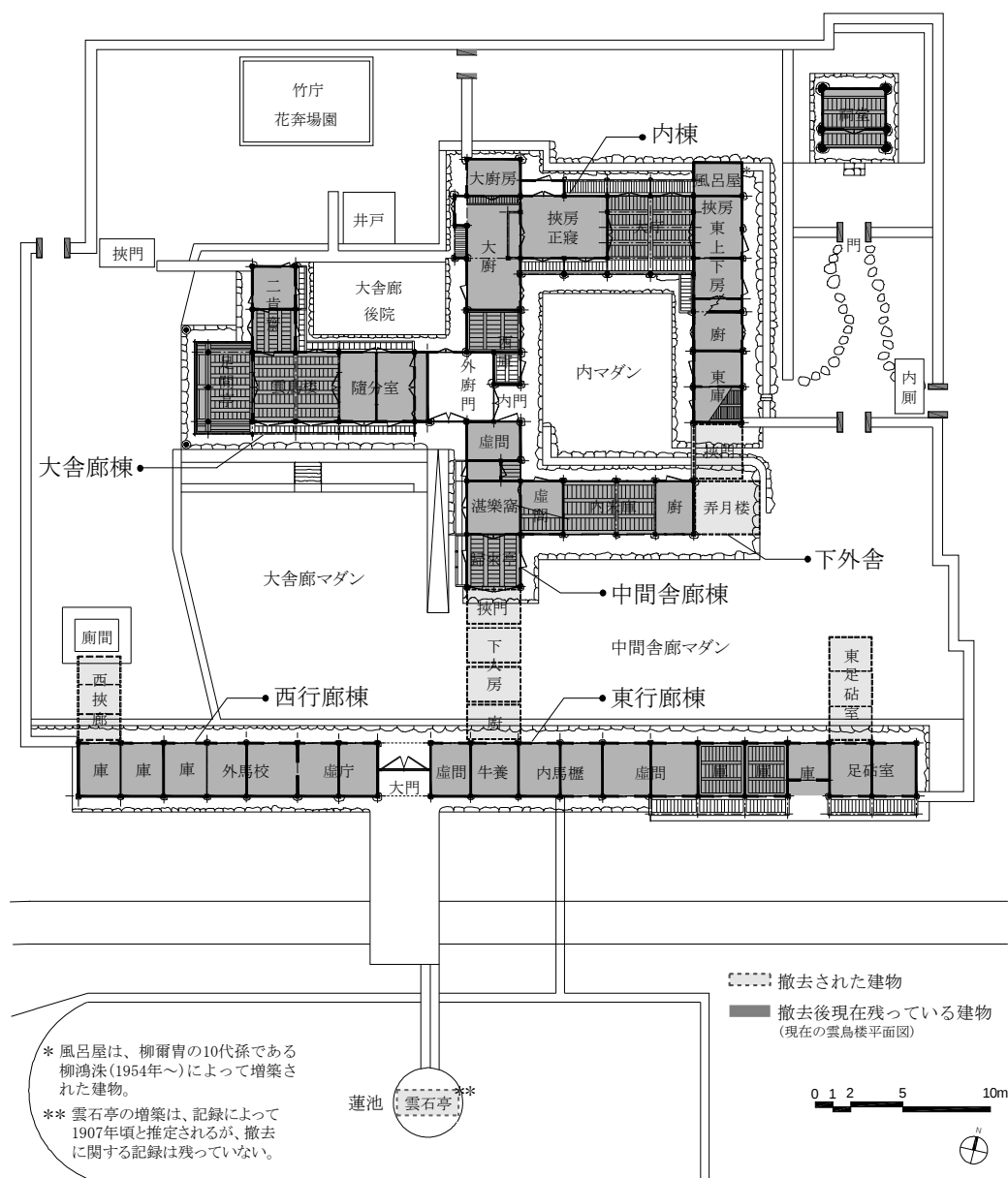
図3 雲鳥楼の平面図
