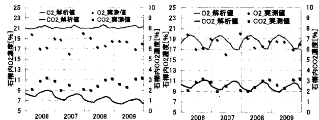
図4 生物活動を考慮しない場合の解析結果
