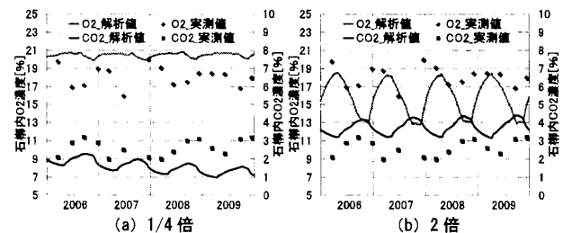
図8 微生物・植物根の酸素消費係数を変化させた場合の解析結果
