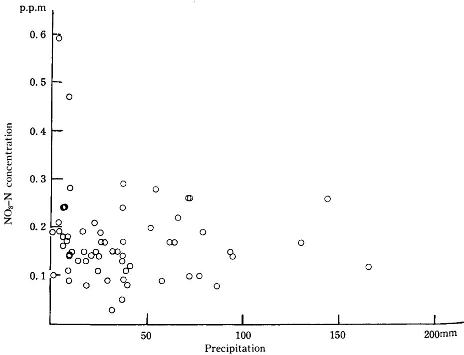
第2図 林外雨の雨量と \text{NO}_3\text{-N} 濃度との関係 Fig. 2 \text{NO}_3\text{-N} concentration and precipitation diagram at open plot.
