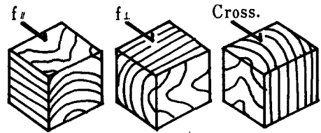
図1 切削方向
