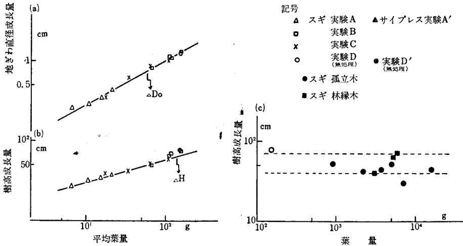
図 2 葉量 ( \bar{w}_L 又は w_L ) と樹高成長量 ( \Delta H ) および地ぎわ直径成長量 ( \Delta D_0 ) の関係 平均葉量 ( \bar{w}_L ) は 1 年前の葉量と現時点での葉量との平均。
