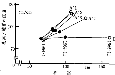
図 11 サイプレス実験の地ぎわ直径に対する樹高の比 ( H/D_0' ) の時間的变化
