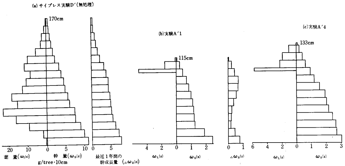
図5 サイプレス実験の葉量，幹量および最近1年間の幹成長量の垂直分布図
