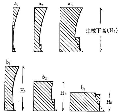
図18 図17から想像される樹冠下での幹成長量の垂直的配分 (a) シリーズは生枝下高が一定で葉量が異なるばあい (b) シリーズは葉量が一定で生枝下高が異なるばあい ただし斜線部は幹成長量を示す
