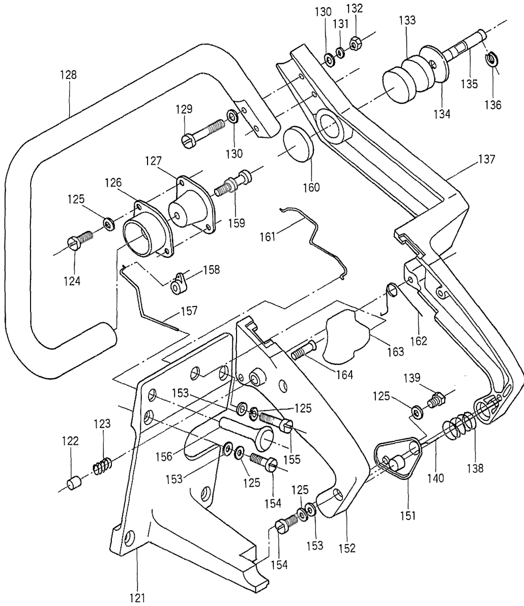
図-2 CH25型チェンソーの防振ハンドル部の構造（取扱説明書より）
