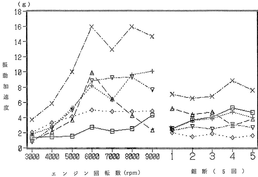
図一4 CH25型の振動加速度 (レーシングと鋸断5回) (図中の記号 □: 前ハンドル前後方向, ◇: 前ハンドル左右方向, +: 前ハンドル上下方向, △: 後ハンドル前後方向, ▽: 後ハンドル左右方向, ×: 後ハンドル上下方向)
