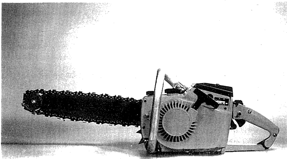
写真一 中国製チェーンソー051型（高把式，藤井裕雄氏撮影）
