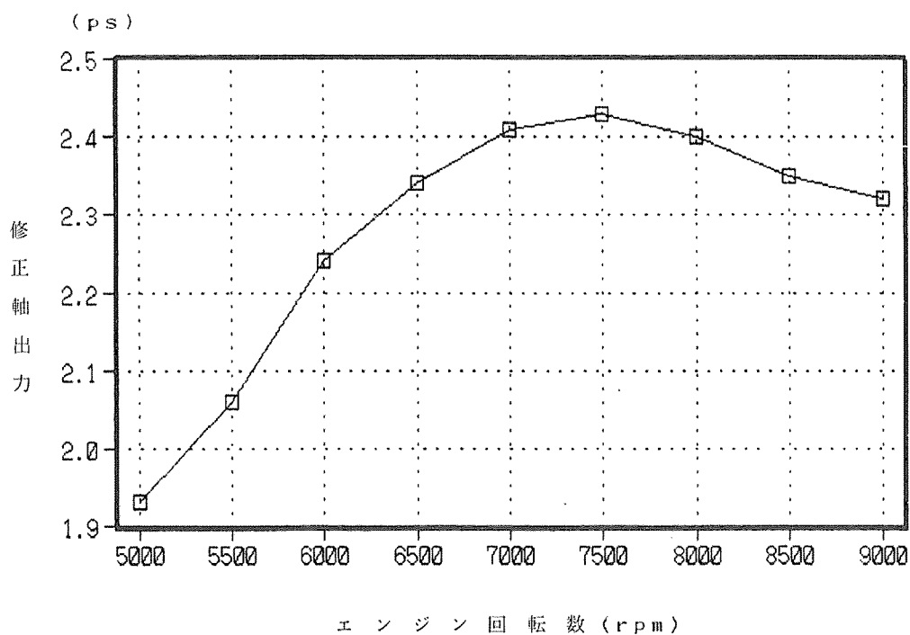
図-6 CH25型の修正軸出力 (遠心クラッチ, ソーチェーン, ガイドバー無し)
