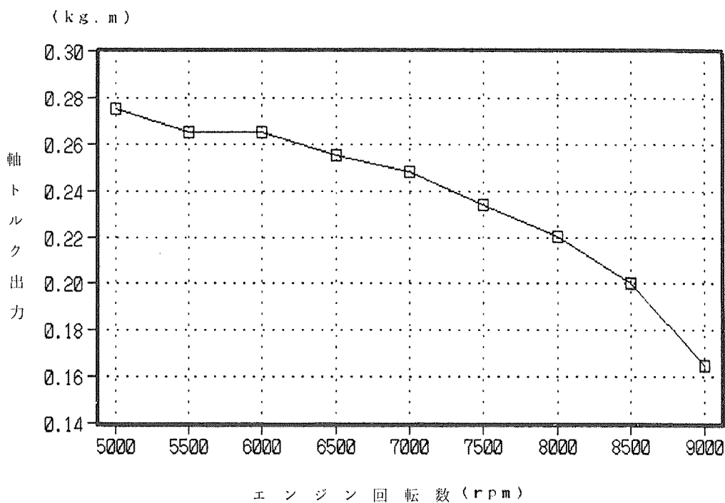
図-7 CH25型の軸トルク出力 (遠心クラッチ, ソーチェーン, ガイドバー無し)
