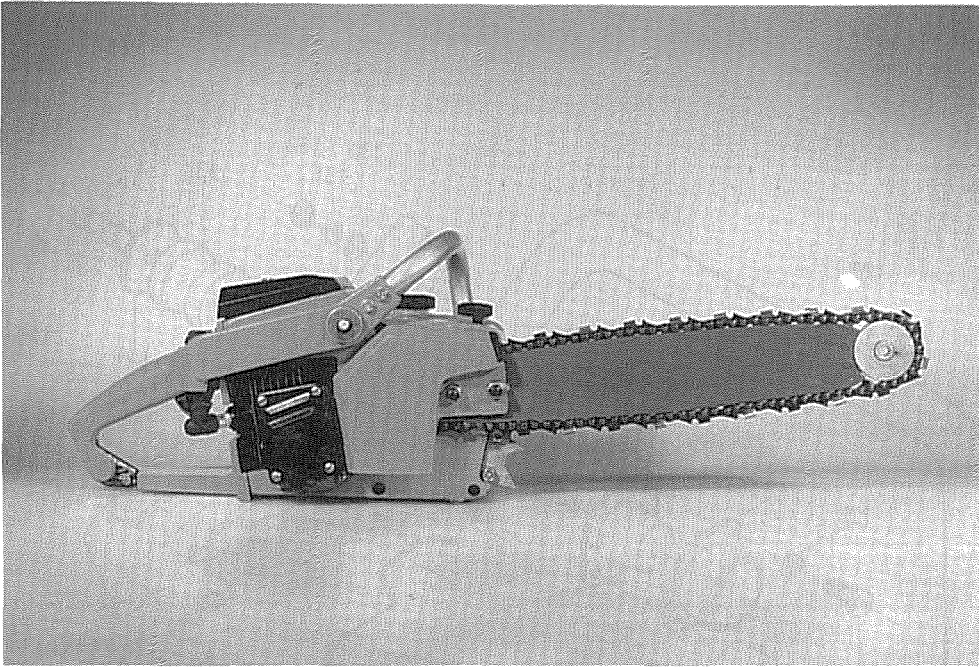
写真-3 CH25型の外観（右側面）
