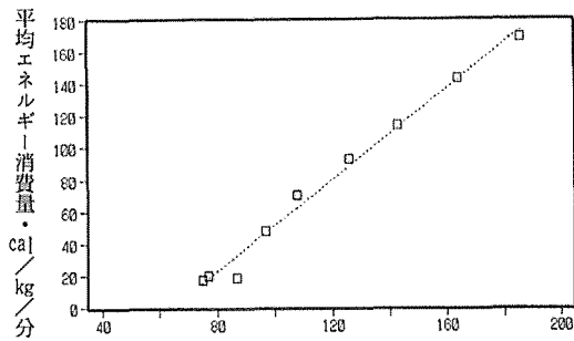
□:測定値 …:計算値 図4 作業者Oの測定値と回帰式 Y=1.4301X-91.77 ( R^2 乗=0.9877)
