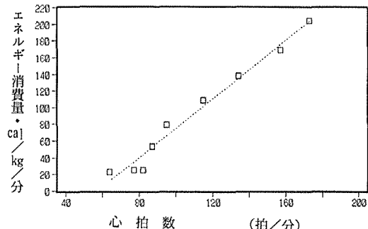
□:測定値 …:計算値 図3 作業者Tの測定値と回帰式 Y=1.7538X-99.89 ( R^2 乗=0.9768)
