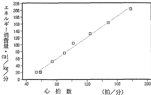
□:測定値 …:計算値 図2 作業者Nの測定値と回帰式 Y=1.5294X-62.67 ( R^2 乗=0.9930)
