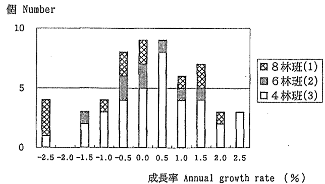
図-3. 広葉樹の成長率の分布
