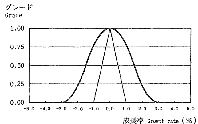
図-4. メンバシップ関数
