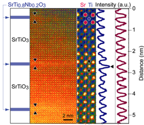
17単位格子の絶縁体SrTiO 3 と1単位格子の金属SrTi 0.8 Nb 0.2 O 3 を交互に積層した人工超格子 = 2次元電子ガス材料
