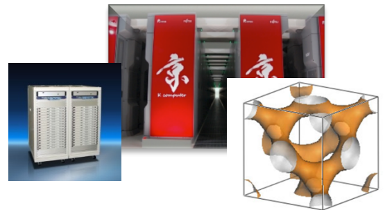
電子構造
