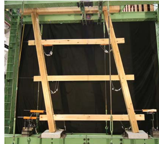
【三段貫】
