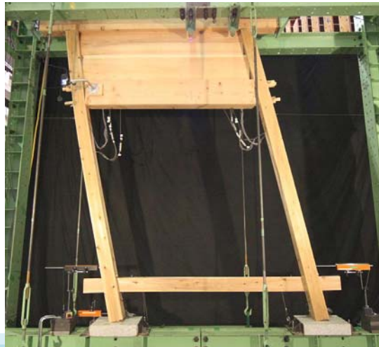
【板垂壁】
