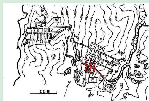
坑道平面図。赤色部分が観測に使用している部分
