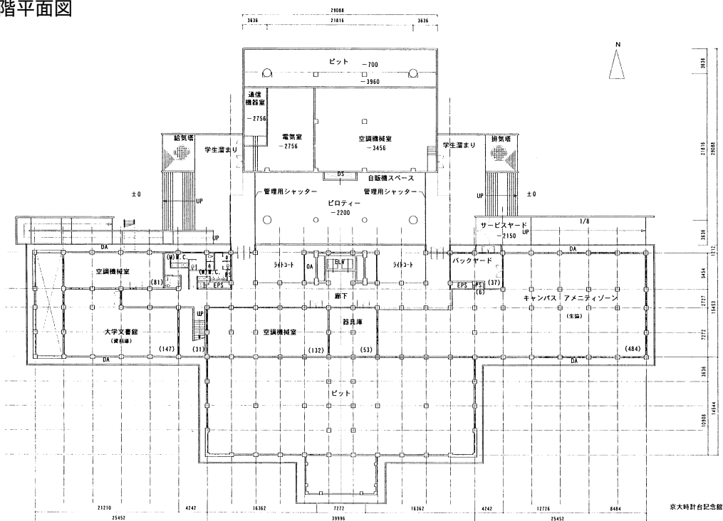
地階平面図
