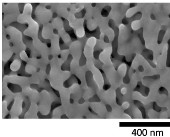
図 1 ナノポーラス金の走査電子顕微鏡写真
