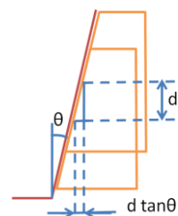
図 4 半径変化量の算出
