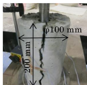
写真 3 載荷後の円柱供試体の様子 (左:ひび割れ状況, 右:内部の状況)
