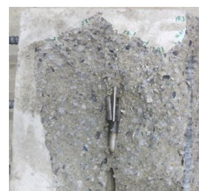
写真 2 載荷後の直方体供試体の様子 (左:表面ひび割れ状況, 右:剥離部分除去後)
