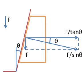
図 3 膨張圧の算出
