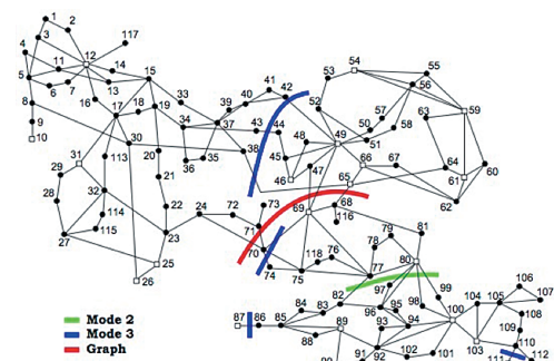
図：Koopman モードに基づく提案アルゴリズムにより得られた IEEE-118 母線モデルの分割[5]。異なる振動モード（時空間変動；Mode2 及び Mode3）により異なる分割が得られる。Graph はグラフラプリアンに基づく従来法で得られた分割を表している。
