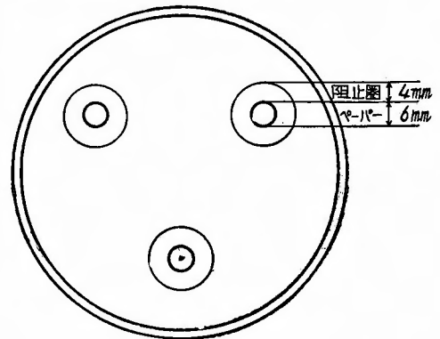
第2図 阻止圏測定法
