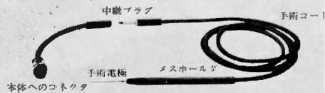
手術電極系の全貌
