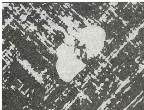
CFRP 積層板の超音波探傷例
