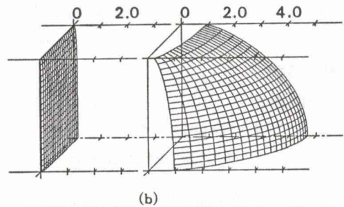
方形断面管を流れる低圧気体の Poiseuille 流 ( U_p ) と熱遷移流 ( U_T ) の流速分布：(a) 高度に希薄な気体、(b) 軽度に希薄な気体
