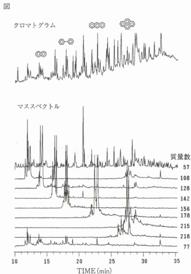
石炭の迅速熱分解により生成した液状物質(タール)のマスキロマトグラムの一例 数多くの化学物質が生成している。
