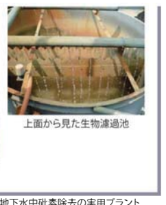
図2:ベトナム農村部に設置した地下水中砒素除去の実用プラント
