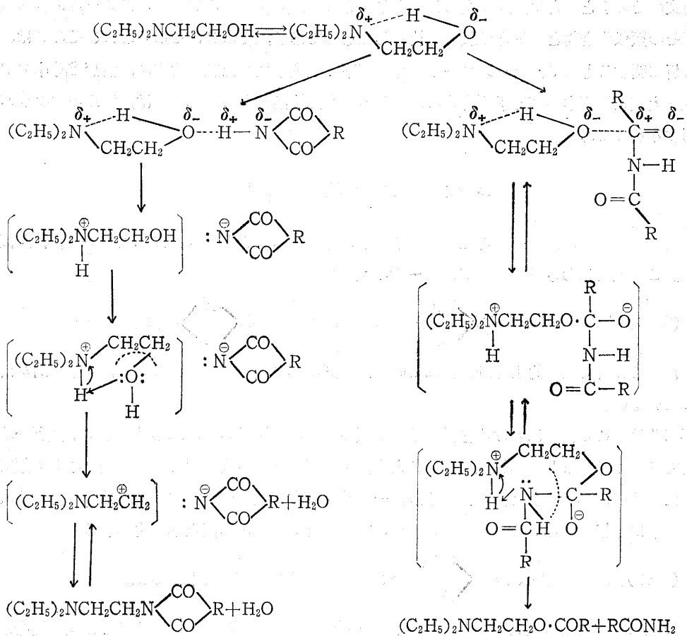
反 応 ( 1 ) 式
