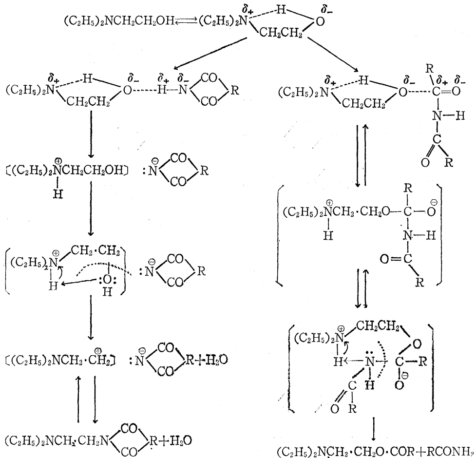
反 応 (1) 式
