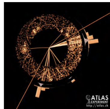
(左) LHC (右) ATLAS 実験 (写真提供: CERN ATLAS 実験グループ) LHC and ATLAS experiment (photo courtesy of CERN ATLAS experiment group)
