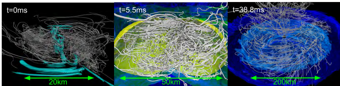
連星中性子星合体が合体しブラックホールと降着円盤およびブラックホール磁気圏が誕生する様子を示した数値相対論的シミュレーションの結果 (Kiuchi et al. 2014)
