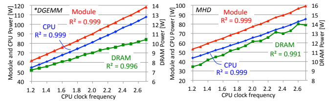
図 4 HA8K の 64 モジュール利用時の消費電力と CPU 動作周波数
