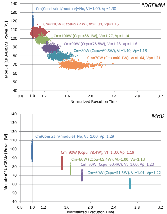
図 2 一律 CPU 電力制約時における実行性能のばらつき
