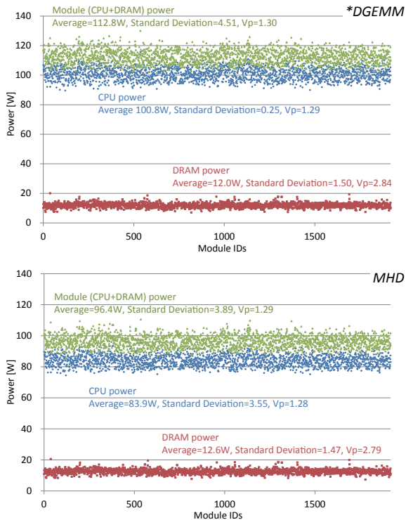
図 1 モジュール消費電力のばらつき
