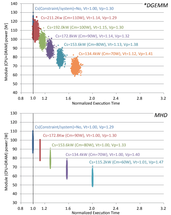
図 8 VaFs 手法における消費電力と性能の詳細
