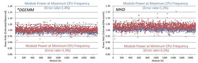
図6 電力推定精度
