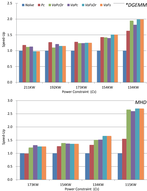
図 7 Naive 手法に対する性能向上比
