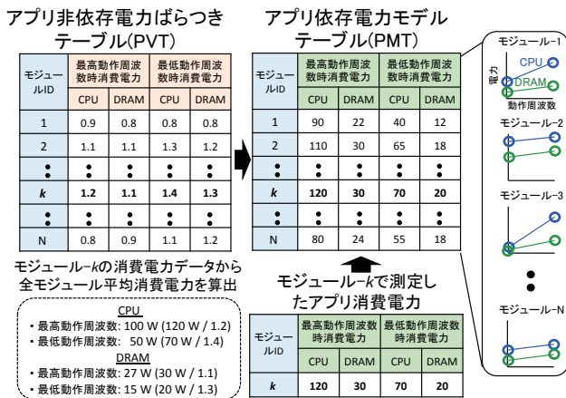
図5 電力モデルキャリブレーション
