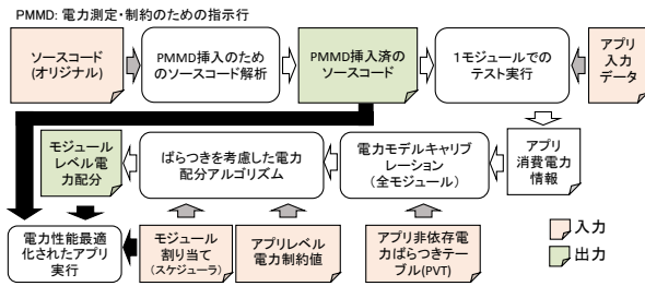
図 3 電力配分のための提案フレームワーク
