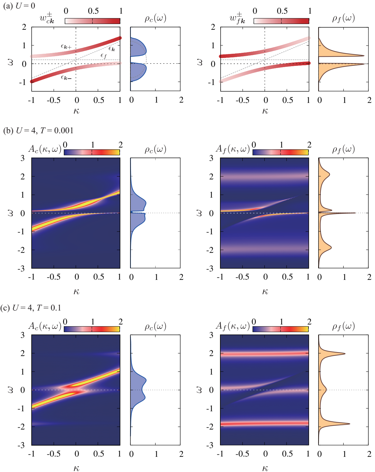
図 14: (a) U=0 の周期アンダーソン模型のエネルギー分散を「波数」 \kappa \equiv \epsilon_{\mathbf{k}} の関数として表した図。左が伝導電子 c、右が f 電子。色の濃さは重み w_{\alpha\mathbf{k}}^\pm を表す。点線は混成がない場合のエネルギー分散。ベーテ格子上の強束縛バンド（状態密度はバンド幅 2D の半円形）を考えている。パラメータは D=1 として、 V^2=0.22 , n=1.9 である。(b),(c) は U=4 の場合の動的平均場理論による一粒子励起スペクトル A_\alpha(\kappa, \omega) と状態密度 \rho_\alpha(\omega) 。ソルバーは CTQMC 法。(b) T=0.001 , (c) T=0.1 。
