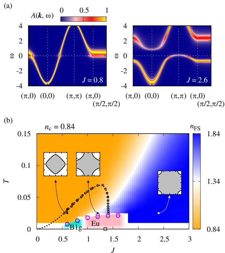
図 21: デュアルフェルミオン法による 2 次元正方格子上の近藤格子模型における (a) 一粒子励起スペクトルと (b) 超伝導相図 [59]。伝導電子数 n_c = 0.84 のハーフフィリング近傍。 B_{1g} と E_u はそれぞれスピン一重項の d_{x^2-y^2} 波と p 波の対称性を持つ超伝導。強度プロットはフェルミ面の囲む体積によって定義される電子数 n_{FS} を表す。丸と点線は反強磁性相の目安を表す (ハーフフィリングの場合)。図は文献 [7] より。
