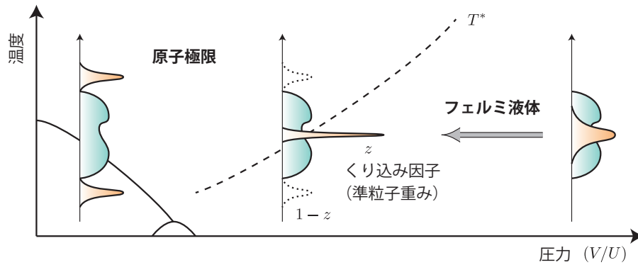
図 7: フェルミ液体論によるアプローチの概念図。破線はフェルミ液体論で到達可能な限界の目安を表す。
