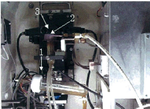
写真-3.5 地盤環境影響物質の微量分析装置；(左)高周波プラズマ発光分析装置による分析。ネブライザ、チェンバ1)より霧化した試料をプラズマ2)内へ導入する。高周波融合プラズマによって試料に電気/熱エネルギーを与えることにより発光させ、放射された光を3)を通して内部の分光器により各元素固有のスペクトル線に分け、スペクトル線の有無と強度から試料中の元素の定性/定量分析を行う。無機汚染物質に適用。(右)ガスクロマトグラフ質量分析計。有機系汚染物質の定性/定量分析
