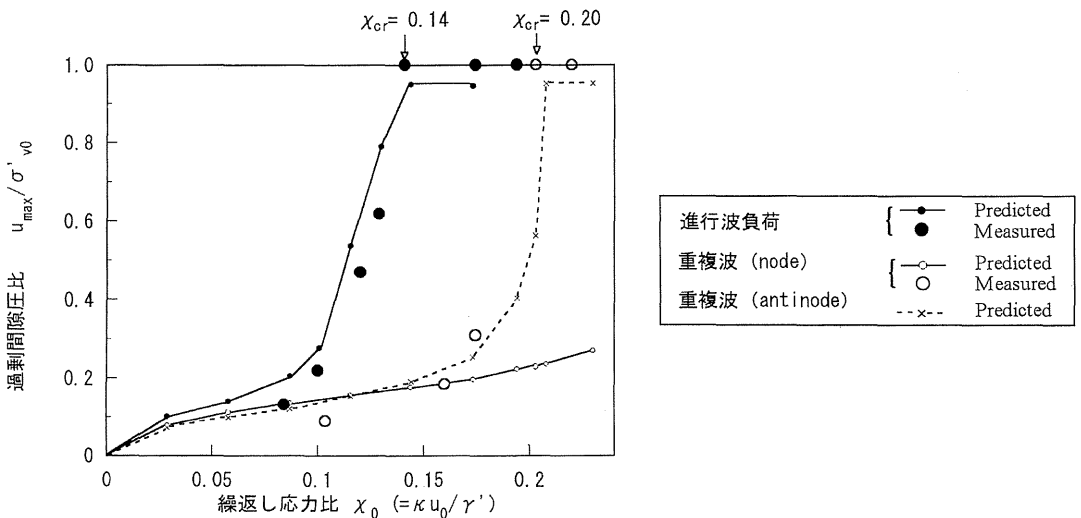
図-3.9 波浪荷重による繰返し応力比と過剰間隙圧比の関係
