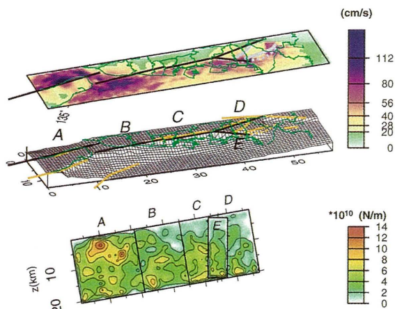
図-3.8 強震動評価の例。1995年兵庫県南部地震の神戸～阪神間の地震動シミュレーション。震源モデル（下段。オレンジ色ほど地震モーメント解放量が大きかった）及び基盤構造モデル（中段）を組み合わせた地震動シミュレーションによって得られた最大水平地動速度分布（上段。濃色ほど大きな地動速度であった）。神戸～阪神間に広がった甚大地震災害域とよく対応している。
