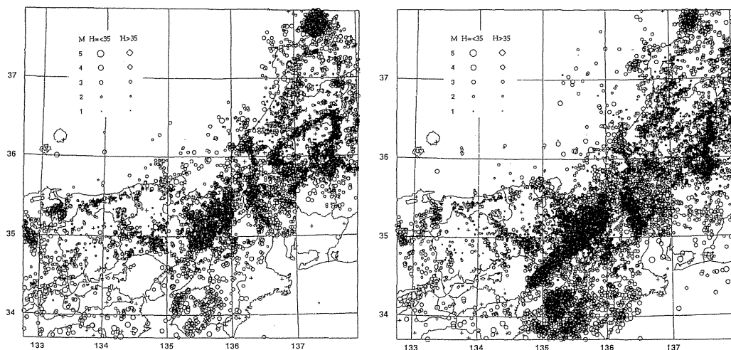
図-3.17 SATARNシステムによる1990年～1998年の西南日本内帯の震央分布図。左は1990年1月1日～1995年1月16日（兵庫県南部地震の前日）、右は1995年1月17日～1998年12月31日を示す。
