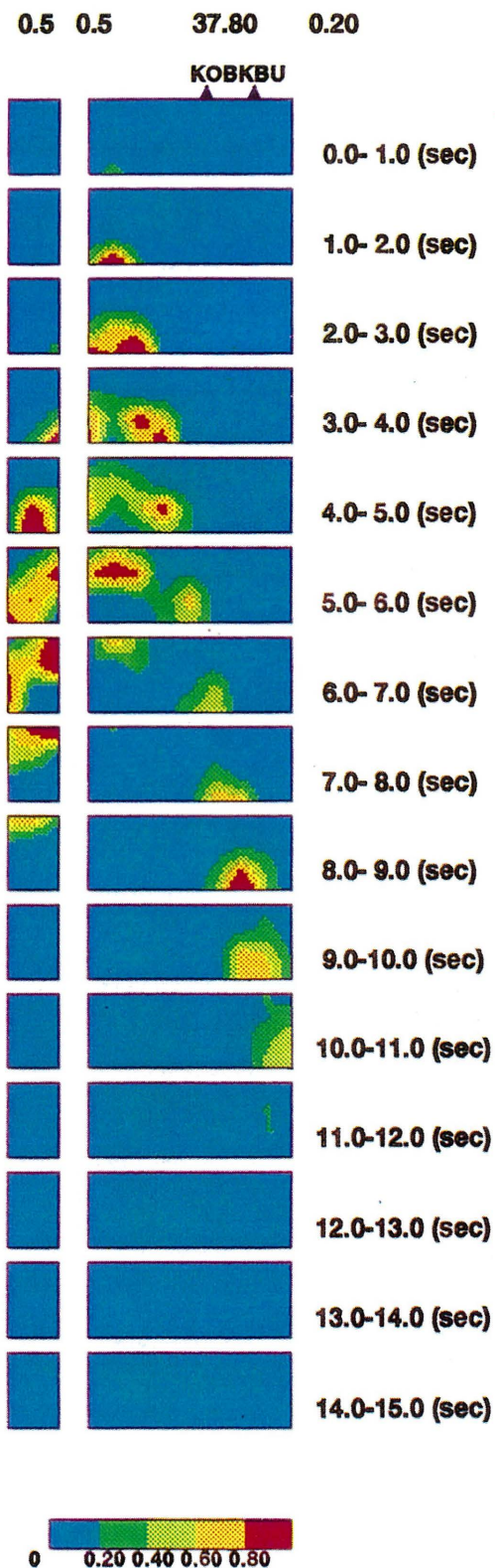
図-3.11 1995年兵庫県南部地震の破壊プロセスのスナップショット
