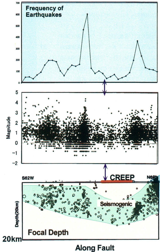
図-3.20 跡津川断層に沿う地震数（上図）、マグニチュード（中図）および地震の深さ分布（下図）クリープの部分で地震数が少なく、Mも小さく、地震は深さ7-17 km で発生するなど他の部分と異なっている。
