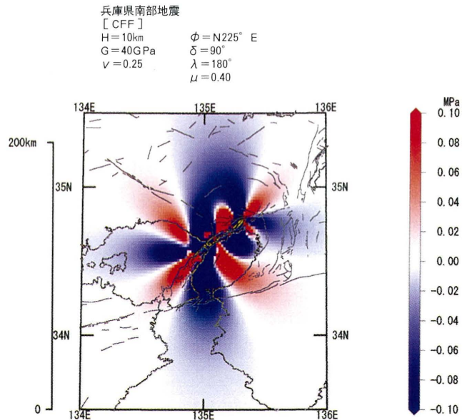
図-3.12 兵庫県南部地震の断層モデルから計算される \Delta CFF の分布
