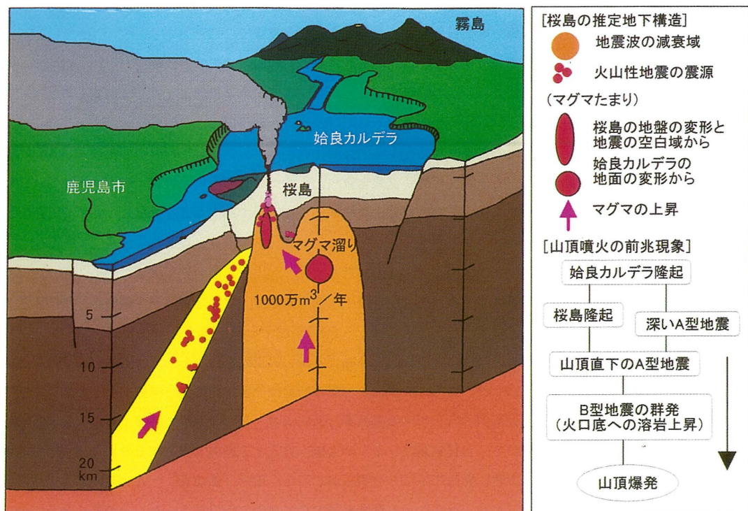
図-3.23 桜島・始良カルデラのマグマ供給系のモデル
