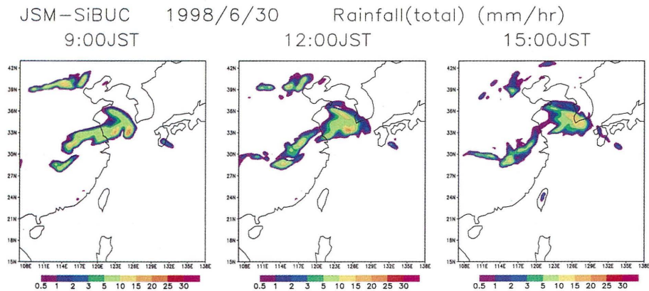
図-3.26 領域気象モデルによる梅雨性降雨のシミュレーション
