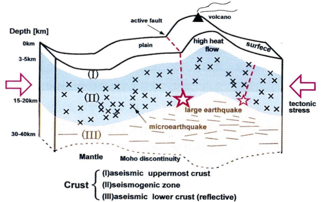
図-3.10 地殻の不均質構造と内陸大地震の核形成のモデル (Ito, 1999)
