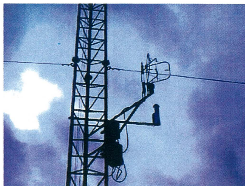
写真-3.15 野外実験場の観測鉄塔の乱流観測機器
