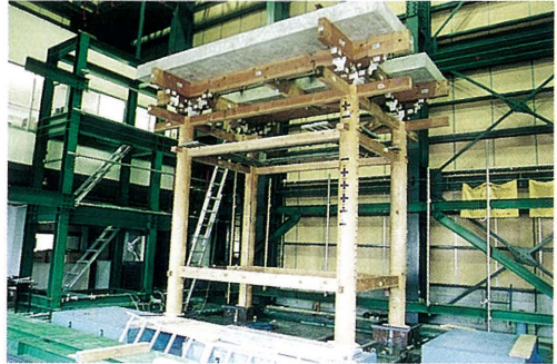
写真-3.4 伝統木造軸組の実大振動実験
