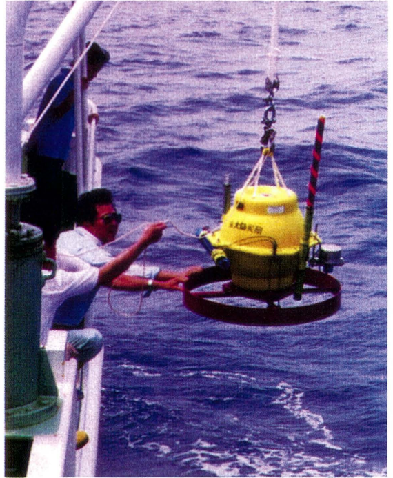
写真-3.22 海底地震計投入作業
