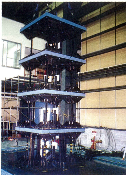
写真-3.28 4層鉄骨造立体骨組の振動台実験
