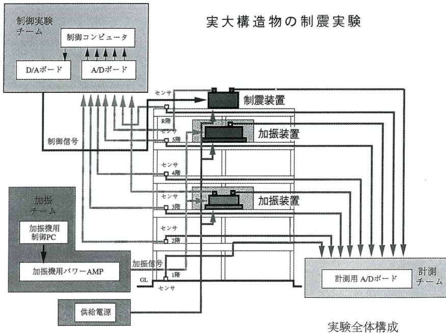
図-3.5 実大構造物の制震実験システム構成
