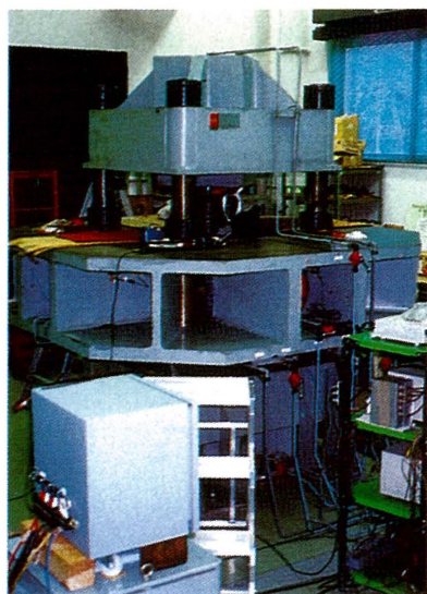
写真-3.21 高温高压岩石破壊実験装置
