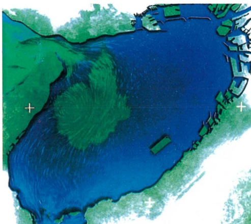
大阪湾の潮流模型実験における流況写真
