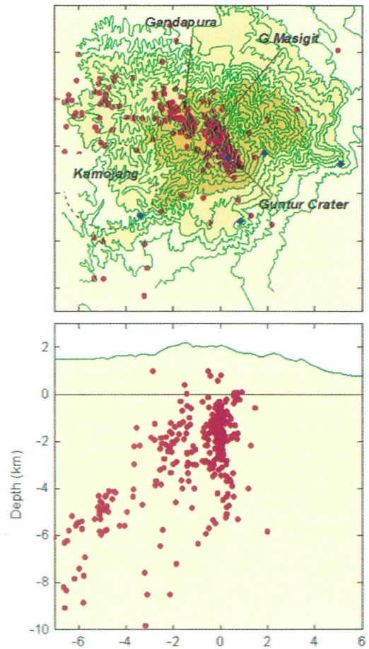
図-3.24 インドネシア・グントールの火山性地震震源分布
