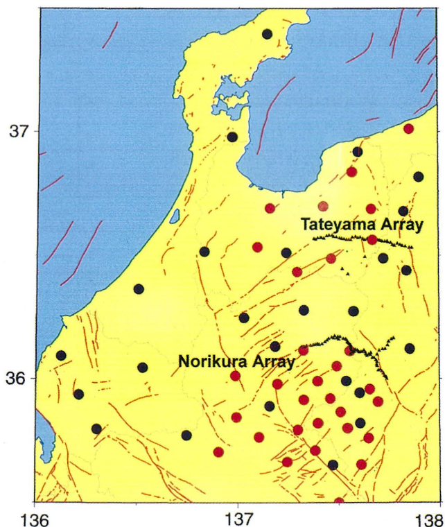
図-3.21 飛騨山地における観測点とアレー観測の図、赤丸は臨時観測点、黒丸は定常観測点、赤い線で活断層を示した。
