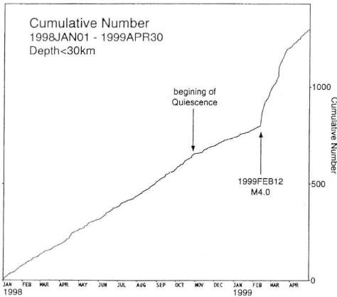
図-3.13 1999年2月12日亀岡付近の地震M4.0を中心とした10km四方の領域内の積算地震発生数
