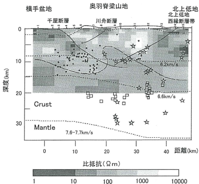
図-3.22 東北脊梁地域を横切る比抵抗構造、破線比抵抗構造の変化を示す。実践は推定された断層面、点線はP波の速度構造の不連続面、●点は微小地震の震源、☆は地震波の反射面、□は低周波地震
