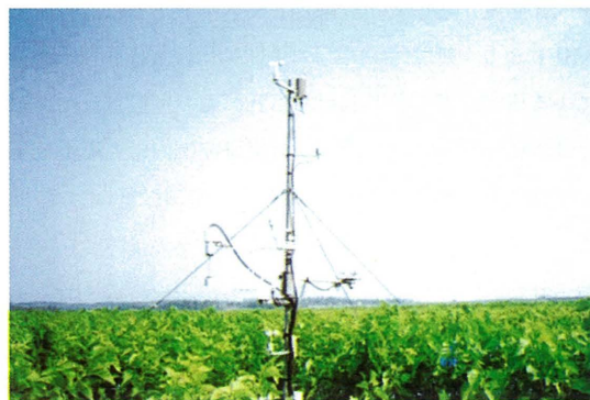
淮河流域の畑地上でのフラックス
