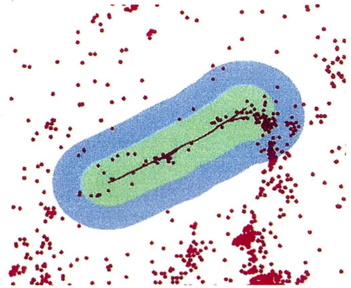
図-3.14 断層からの距離による領域分けに震央を重ねる方法の模式図
