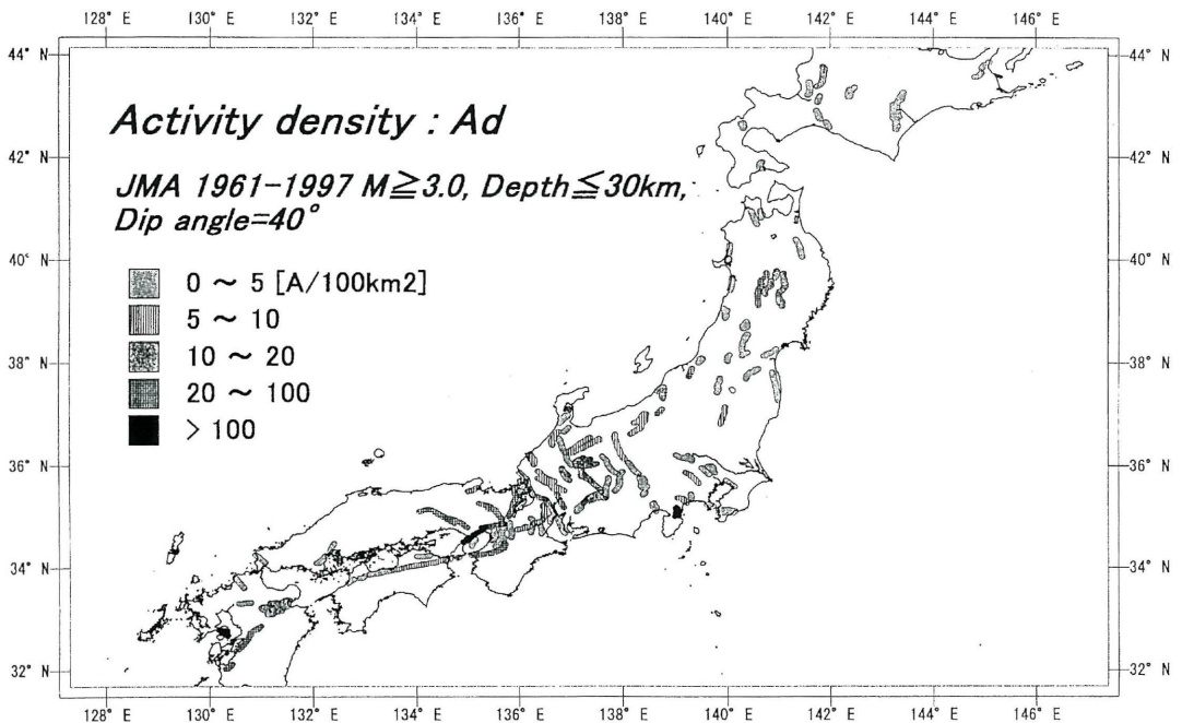
図-3.15 全国の活断層（推進本部の調査98断層）に関する地震活動度（Tsukuda,1985）密度の分布。関東、東北に低く中部、関西に高いことが判る。
