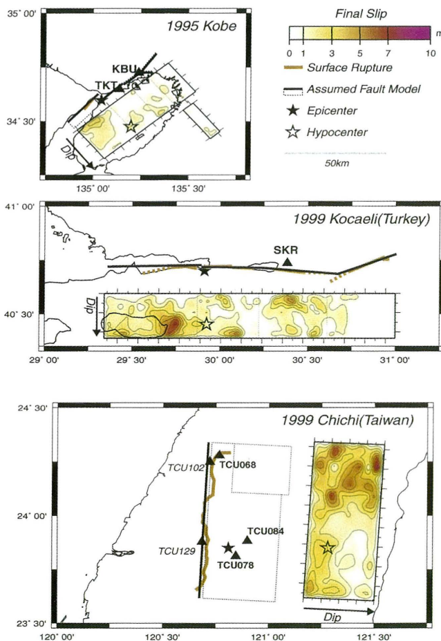
図-3.7 強震動記録を用いた断層破壊過程の推定例。1995年兵庫県南部地震，1999年トルコ・コジャエリ地震，台湾・集集地震の断層モデルと断層面上での最終すべり分布を示している。星印は発震点。断層地震規模の違いと断層すべりの不均質性が見られる。
