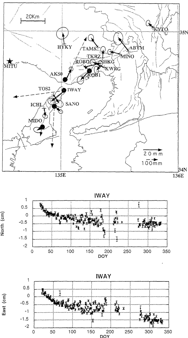
図-3.18 GPSによる兵庫県南部地震の余効変動：(上) 水平変動場 (実線)。破線は地震時の変動。(下) 岩屋の変位の時間変化。
