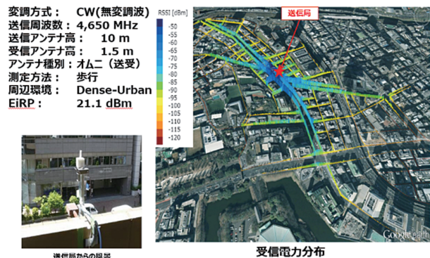
図9：都市部における4.5GHz伝搬実験の様子
