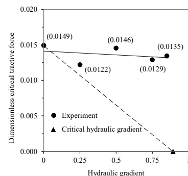
動水勾配と限界掃流力の関係
