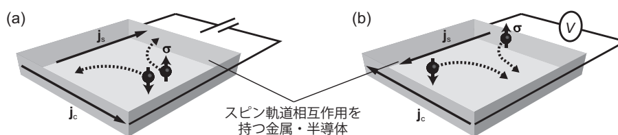
図 3 (a) スピンホール効果 (電流→スピン流変換) の模式図。(b) 逆スピンホール効果 (スピン流→電流変換) の模式図。
