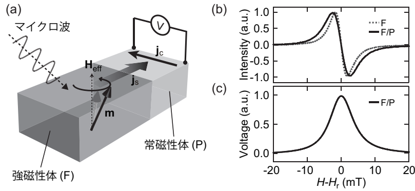
図4 (a) 強磁性体 (F)/常磁性体 (P) 接合におけるマイクロ波誘起スピンプングの模式図。FMR 条件下で生成されたスピンプングが逆スピンプング効果によって電流に変換される。通常は開回路条件で電圧信号として測定する。(b) F 単層薄膜及び F/P 二層薄膜におけるマイクロ波吸収スペクトルの例。(c) F/P 二層薄膜における起電力の磁場依存性。F 層が FMR 条件を満たした際に大きな起電力信号が観測される。 H は外部磁場強度、 H_r は共鳴磁場である。
