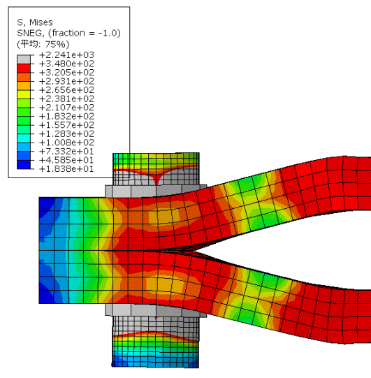
(b) 終局時の引張接合部の変形状
