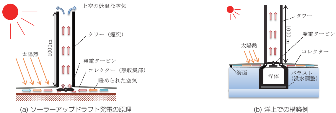
図-7 洋上でのソーラーアップドラフト発電の概念
