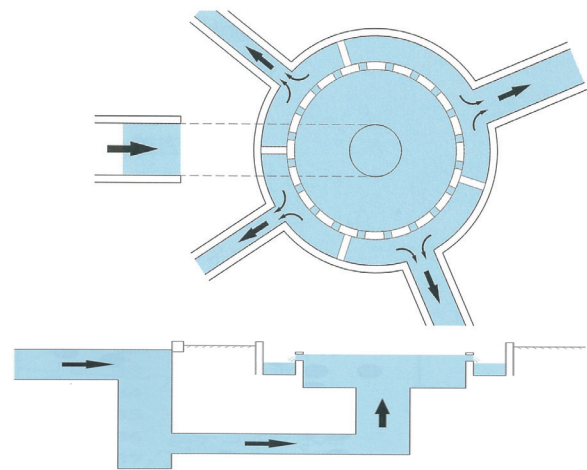
図-1 角度の概念の理解と逆サイホンの原理
