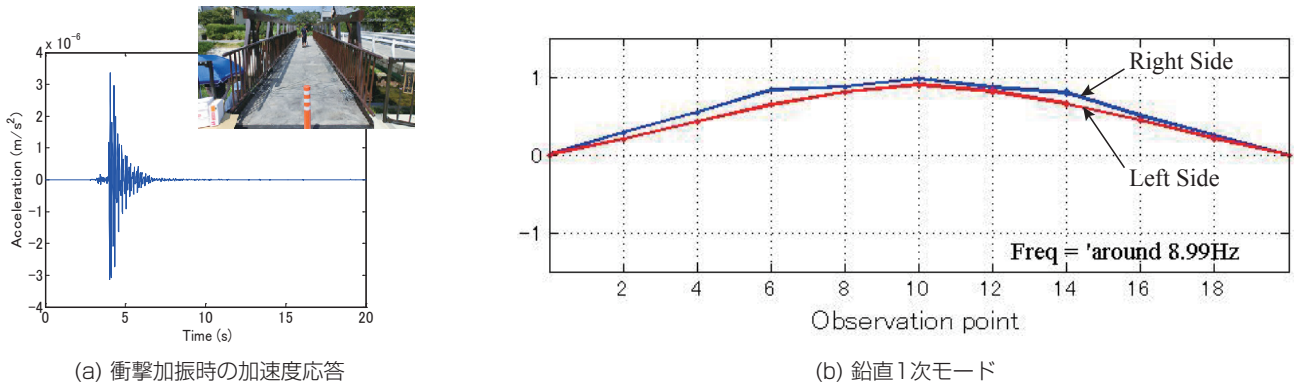
図-5 FRP歩道橋における振動計測
