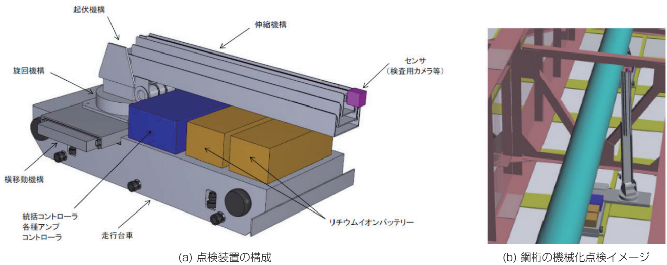
図-6 桁橋の機械化点検の概念図
