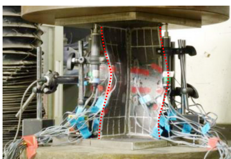
(a) 十字断面柱の座屈実験
