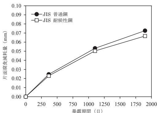
(a) 中国・上海市における鋼材の腐食進展
