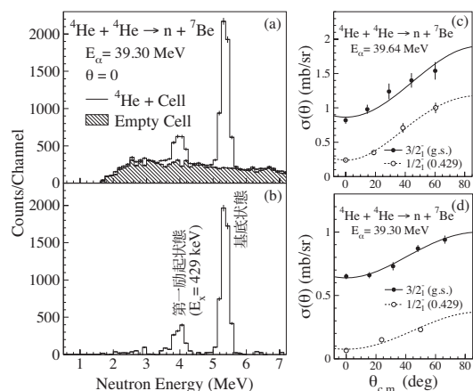
図 5 (a) {}^4\text{He} + {}^4\text{He} \rightarrow n + {}^7\text{Be} 反応における中性子のエネルギースペクトル。白抜きと斜線のスペクトルは、それぞれ {}^4\text{He} ガス標的とガスを封入しない標的容器を用いた測定結果。(b) {}^4\text{He} ガス標的のスペクトルからガスを封入しない標的容器のスペクトルを除去したバックグラウンドを除去した中性子のエネルギースペクトル。(c) E_\alpha = 39.64 MeV における {}^4\text{He} + {}^4\text{He} \rightarrow n + {}^7\text{Be} 反応の微分断面積の角度分布。黒丸と白丸はそれぞれ、 {}^7\text{Be} の基底状態と第一励起状態に対する微分断面積を表す。実線と破線は、偶数次のルジャンドル多項式を用いたフィット関数を示す。(d) (c) に同じ。ただし、ビームエネルギーは E_\alpha = 39.30 MeV。
