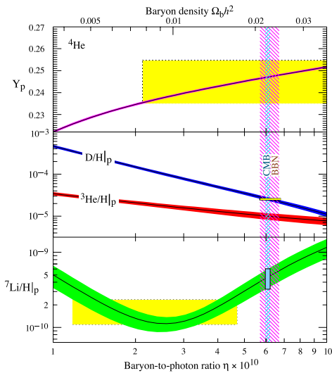
図3 標準ビッグバン模型にもとづく 4 He, 重陽子(D), 3 He, 7 Liの生成量の予測値。横軸は、上がバリオン密度( \Omega_b h^2 )、下がバリオン/光子比( \eta )。 4 Heについては質量存在比( Y_p )、その他の元素については水素に対する個数比で示す。 Y_p , D/H|_p , {}^3\text{He}/H|_p , {}^7\text{Li}/H|_p に現れる添字のpは宇宙の原始(primitive)生成量であることを表す。黄色の四角は、宇宙初期における元素存在量の観測推定値の95%信頼区間と、その推定値から許容される \eta の範囲を示す。斜線で示す縦方向の狭いバンドと広いバンドは、それぞれ、宇宙背景放射(CMB)の観測とビッグバン元素合成(BBN)における重陽子生成量の観測推定値によって制限された \eta の範囲を示す。水色の四角は、BBN計算と \eta から制限される 7 Liの生成量の理論予測値の95%信頼区間を示す。文献 3) の図24.1を一部改変。
