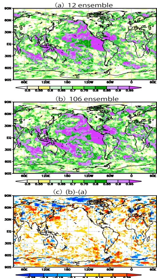
図 2: (a)7-8 月平均の地上 2m 気温偏差を 6 月初旬から予測した場合の、10% tecilies の正イベントの ROC スコアスキル。0.5 以下は精度無しで、1 に近い程精度が高い。解析期間は 1983-2015 年。(a) オペーション化した F2-3DVAR の 12 アンサンブルの結果。(b) LAF によりアンサンブル数を 108 に増やし
