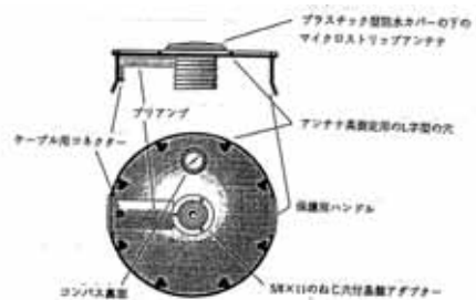
図 4. アンテナ・プラットフォーム (側面図および底面図)
