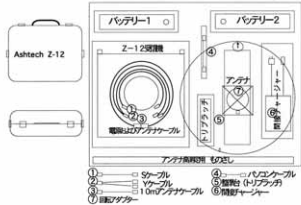
図9 機材の名称と配置図
