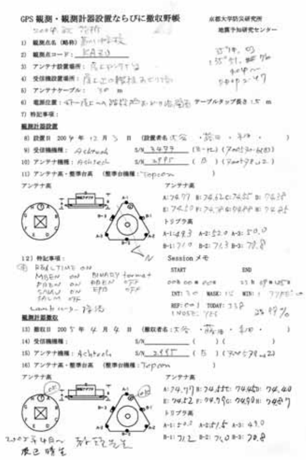
図 14 観測野帳
