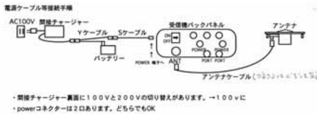
図10 機材配線図
