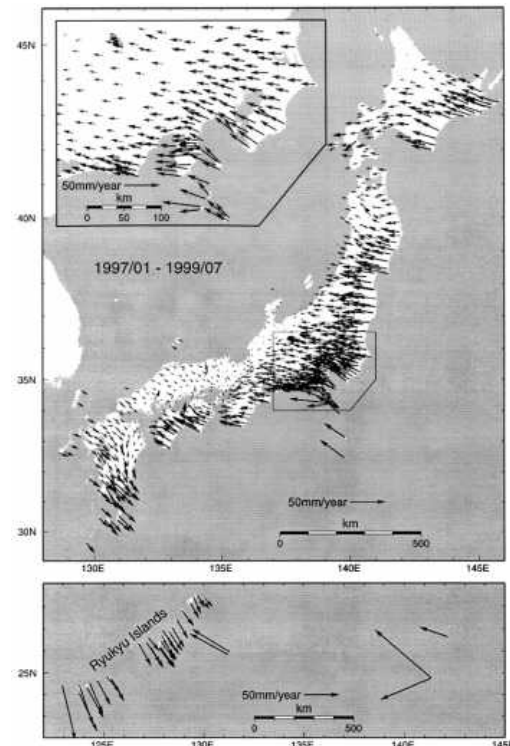
図 2 国土地理院 GEONET による地殻ひずみ
