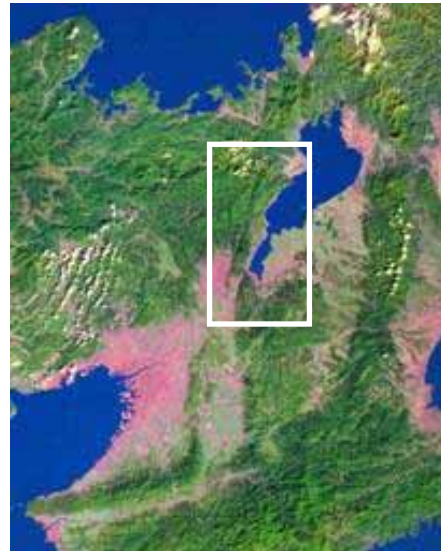
写真 1 花折断層とその周辺 (白枠観測地域)
