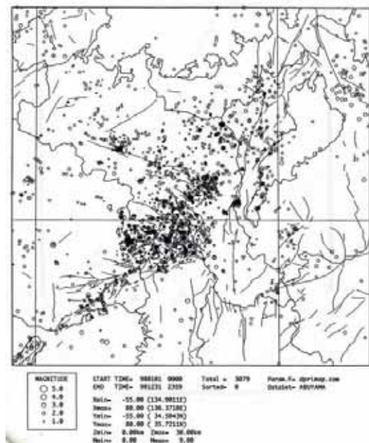
図 3 丹波山地の地震活動 (1998, 1/1-12/31)
