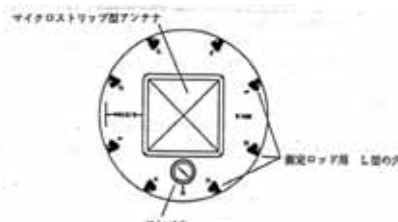
図 3. 精密アンテナプラットフォーム (上面図)
