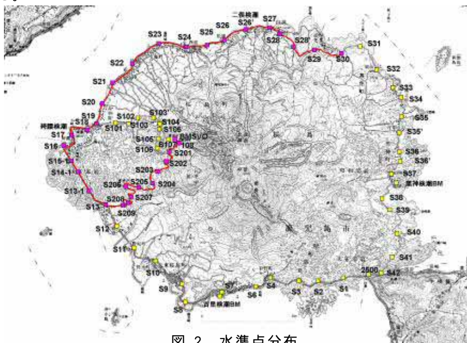
図2 水準点分布
